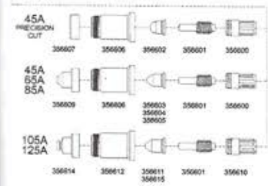
Torcia automatica Machine torch Maschinenbrenner Torche automatique
