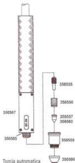
Torcia automatica Machine torch Maschinenbrenner Torche automatique
