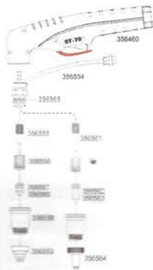
Torcia manuale Hand torch Handbrenner Torche manuelle
